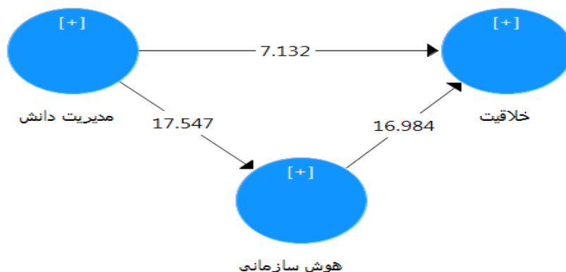
شکل ۵. مدل نهایی پژوهش با مقادیر t
